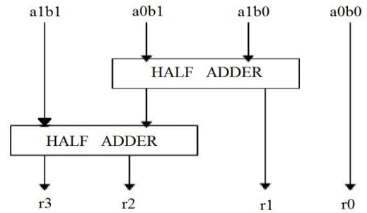
Fig.4. Block diagram 2x2 Vedic multiplier.
